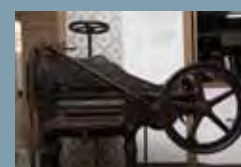
Guilhotina para cortar e aparar papel, cartão, livros e blocos. Foi fabricada na Alemanha por Mansfeld Leipzig Foundry, em 1916. Funciona por accionamento de pedal EMS.2010.00127.00000
